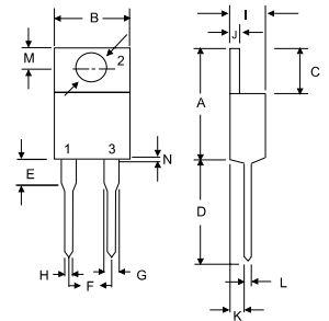
TO-220A
